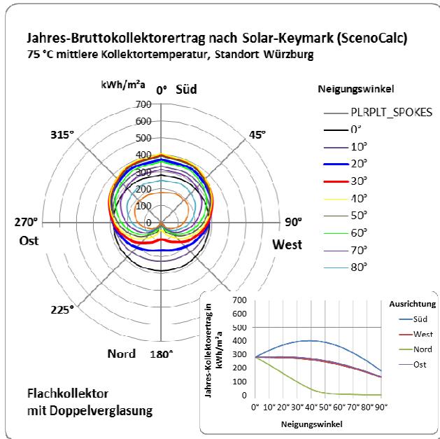
Abb. 8: Kollektorertrag, Richtung und Neigung für einen Flachkollektor mit Doppelverglasung
