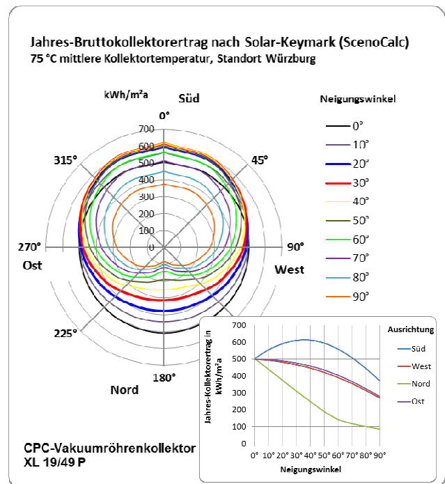
Abb. 7: Kollektorertrag, Richtung und Neigung
