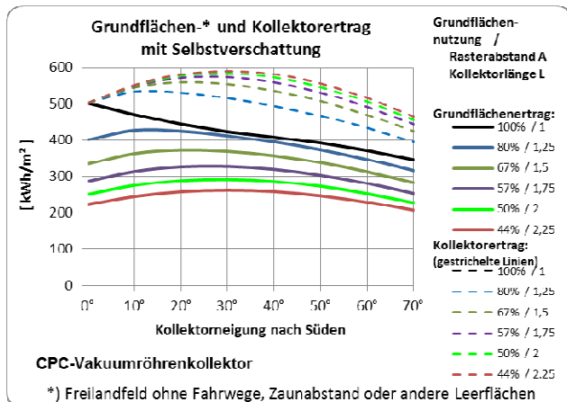
Abb. 13: Grundflächen- und Kollektor-ertrag bei Südnei-gung und verschiedener Grundflächennutzung (CPC-VRK)
