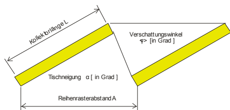
Abb. 9: Kollektorlänge und -Reihenrasterabstand Der Neigungswinkel ist fix, der Verschattungswinkel ist an der Kollektoroberkante Null und wächst nach unten.
