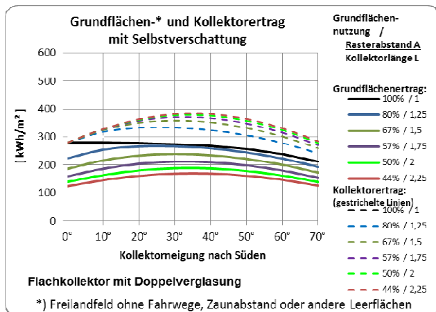
Abb. 14: Grundflächen- und Kollektor-ertrag bei Südnei-gung und verschiedener Grundflächennutzung (Flachkoll.)
