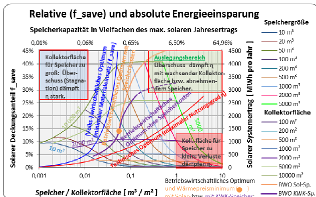
Abb. 1: Die Energieeinsparung in Abhängigkeit vom spezifischen Speichervolumen (vgl. Abb. 6 in Teil 1)
