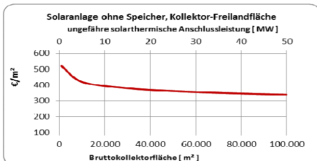
Abb. 4: Kosten Solaranlage ohne Speicher (Freiland)
