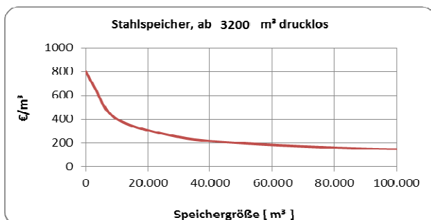
Abb. 5: Kosten Stahlspeicher, drucklos ab 3200 m 3
