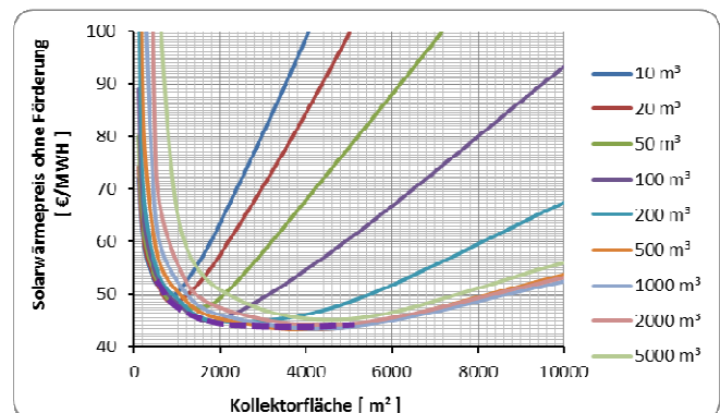
Abb. 3: Solarwärmepreis ohne Speicherkosten
