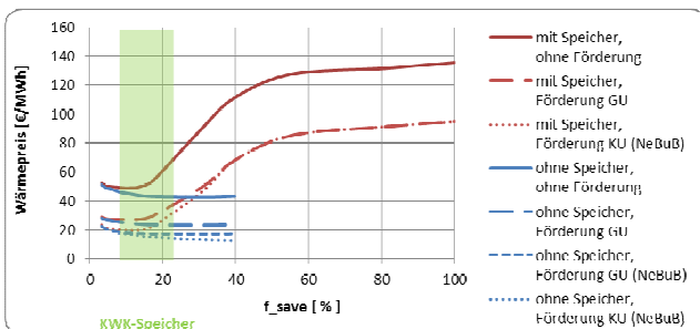
Abb. 8: Wärmepreise mit und ohne Speicher sowie mit und ohne Förderung
