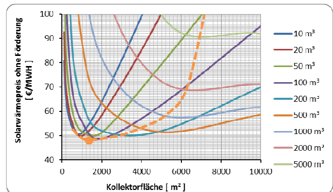
Abb. 2: Solarwärmepreis mit Speicherkosten
