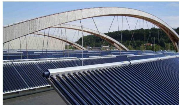
Abb. 11: Dezentrale solare Fernwärme in Wels (A)
