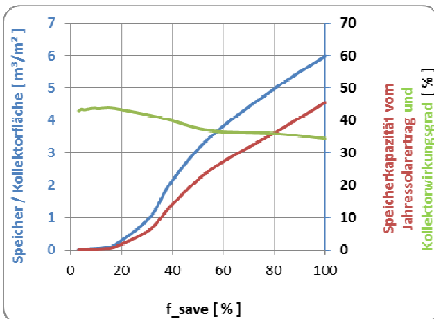
Abb. 7: Spezifische Speichergröße, Speicherkapazität und Kollektorwirkungsgrad mit wachsendem f_{\text{save}}
