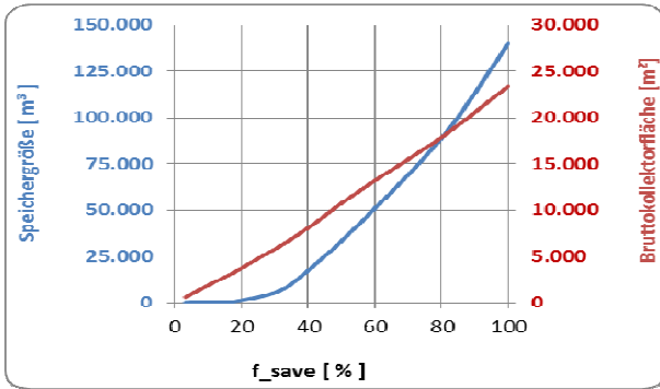
Abb. 6: Bruttokollektorfläche und Speichergröße mit wachsendem f_{\text{save}}
