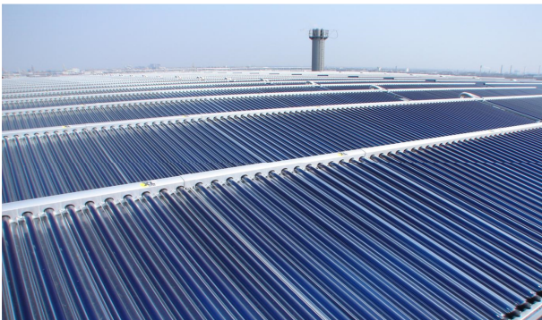
Abb. 9: Zentrale solare FW „Energiebunker Hamburg“
