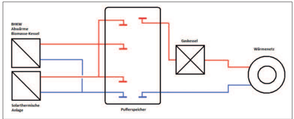
▲ Bild 2 • Anlagenschema EBW
