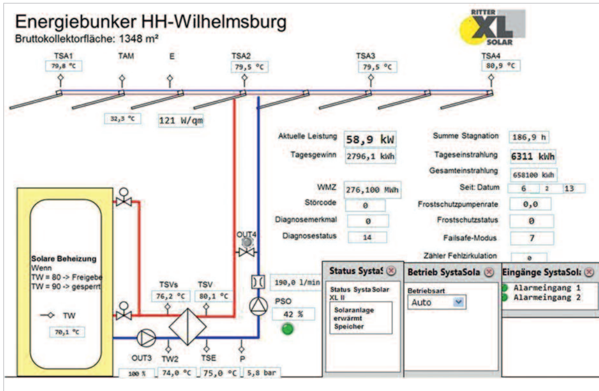
▲ Bild 3 • Anlagenschema EBW (01.08.2013 nach Sonnenuntergang)
