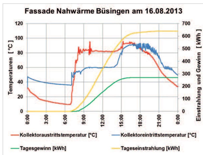
◀ Bild 7 • Fassa- denanlage in Büsing am 16.08.2013
